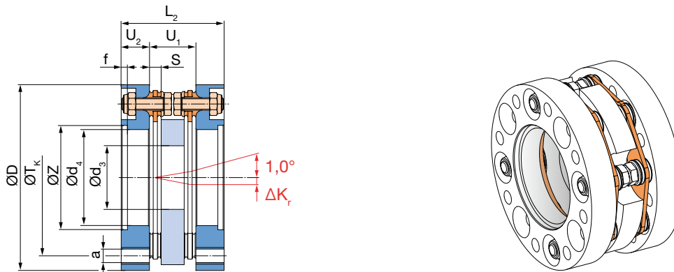
Fig. 69: Type 951.661
