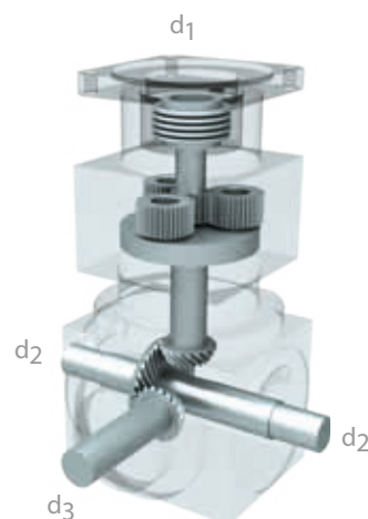
1 zusätzlicher Wellenzapfen ZA 1 additional auxiliary shaft extension ZA
