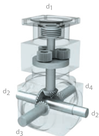
2 zusätzliche Wellenzapfen ZA 2 additional auxiliary shaft extension ZA
