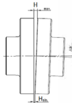
Allineamento angolare Angular displacement
