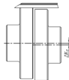
Allineamento radiale / parallelo Radial/parallel displacement
